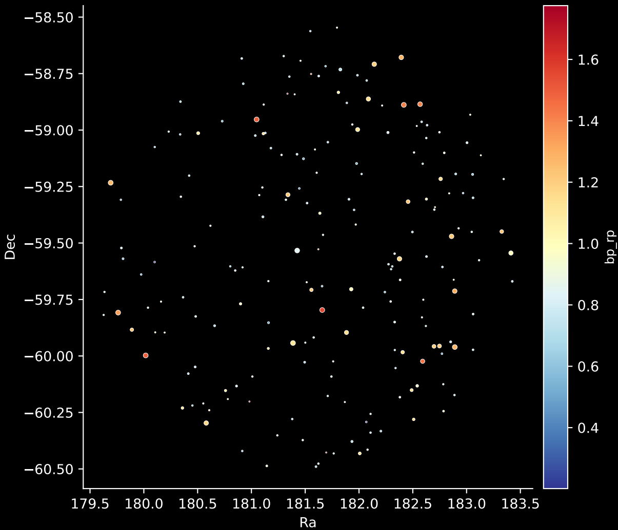
GALAH DR4 Field: [7158] Stars: 196
