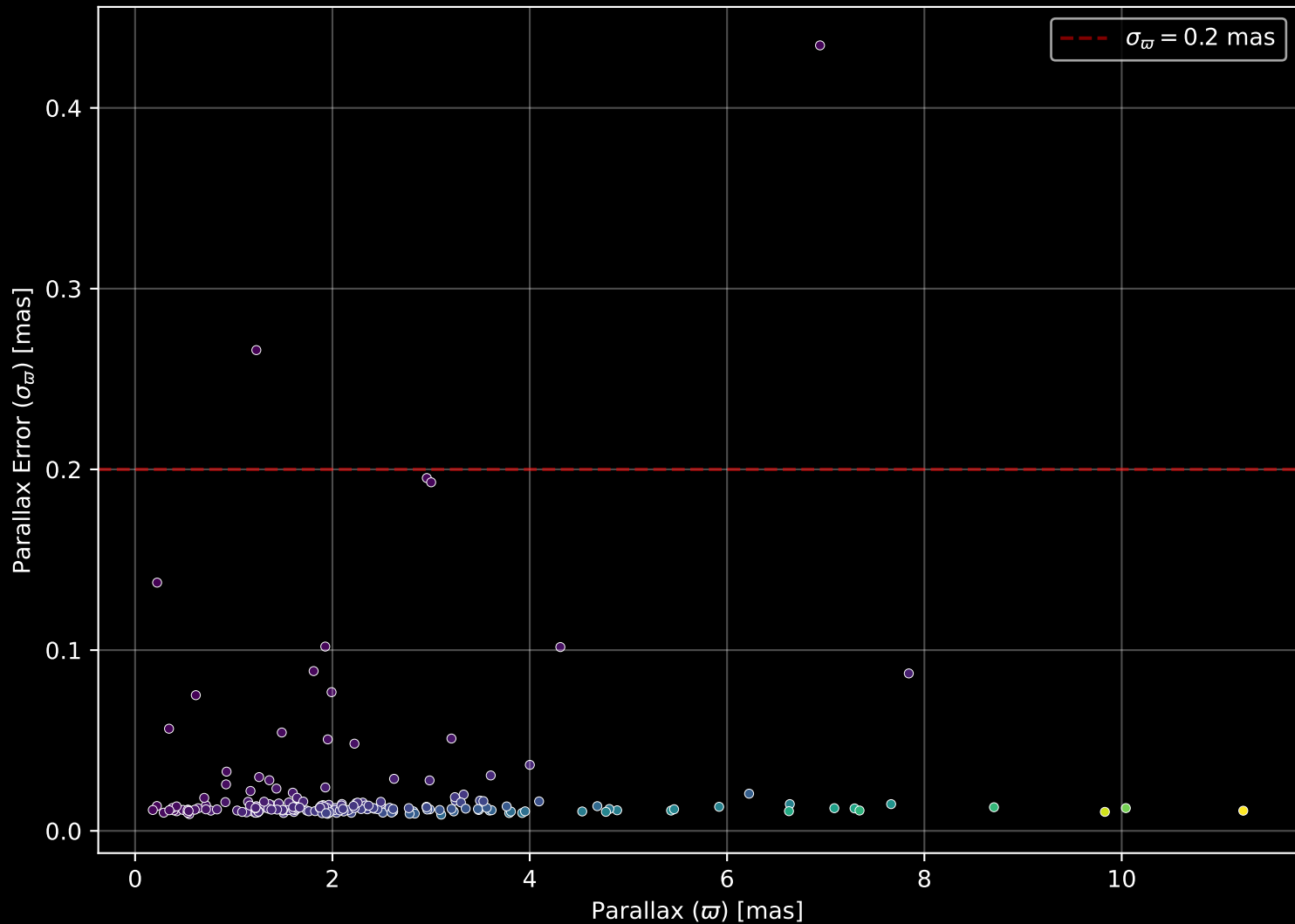
GALAH DR4 Field: [7158] Parallax Quality (n= 196)
