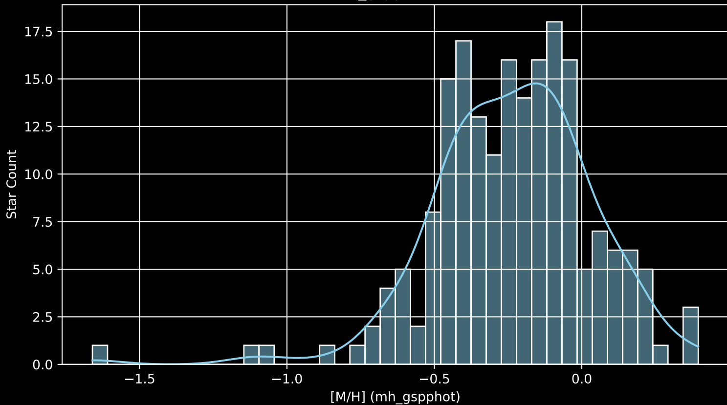
GALAH DR4 Field: [7158] [M/H] (mh_gspphot) (n= 195)
